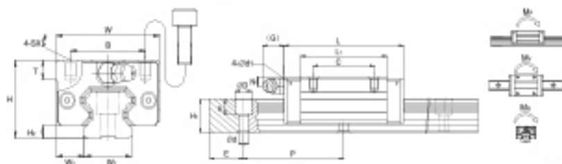
LSA-R/LSA-LR尺寸表
